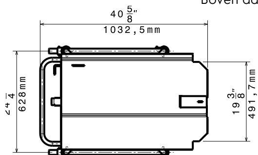
Boven aanzicht
