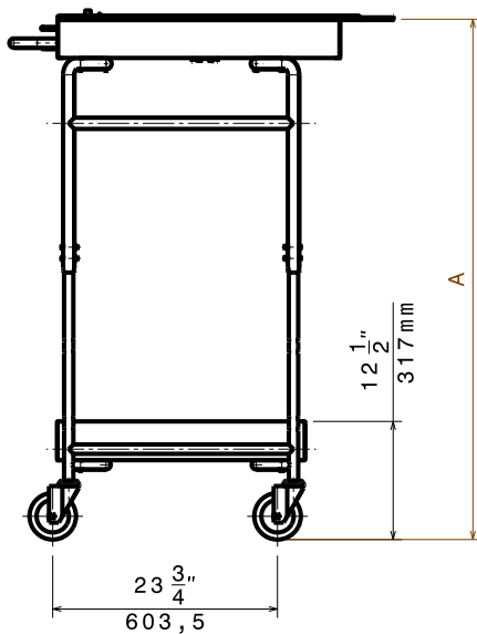
Front aanzicht
